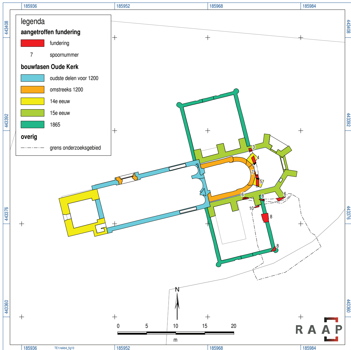
Figuur 10. Aangetroffen funderingen op vlak 1 en vlak 2 geprojecteerd op de gedigitaliseerde tekening van de verschillende bouwfasen van de Oude Kerk (naar Glazema, 1949).
